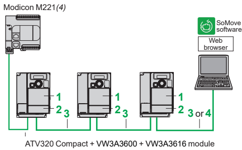
ATV320 Compact + VW3A3600 + VW3A3616 module
