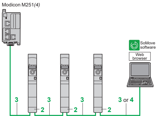
ATV320 Book + VW3A3616 module
